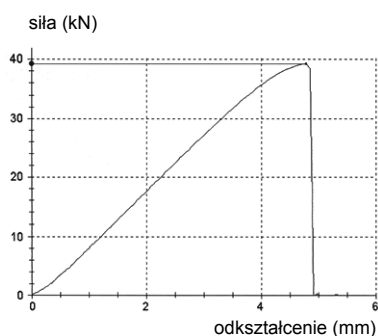
złącze odkuwane
