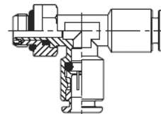
Przyłącze trójnik „L”, gwint zewnętrzny
