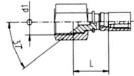
Końcówka z GW, JIC
