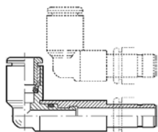
Przyłącze kątowe z króćcem wydłużone, tworzywo
