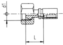
Końcówka z GW, DKL
