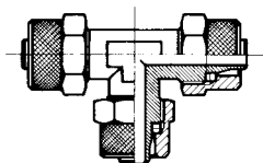
Złącze trójnik
