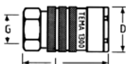
gniazdo z gwintem wewnętrznym
