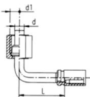
Końcówka 90° z GW z pierścieniem zacinającym, stożek 24°
