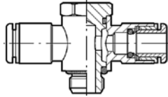
Kompletny trójnik BANJO, mosiądz
