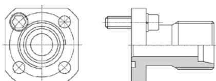
Przyłącze kołnierzowe 4-otworowe / DIN 2353
