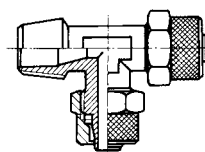
Przyłącze trójnik „L”, gwint zewnętrzny stożkowy
