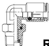
Przyłącze kątowe obrotowe, gwint zewnętrzny stożkowy
