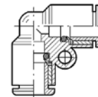
Złącze kątowe przelotowe, tworzywo
