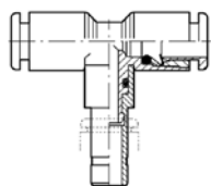
Przyłącze trójnik „T” z króćcem, tworzywo
