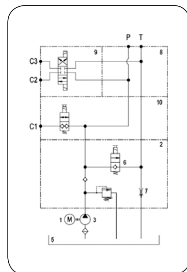
schemat hydrauliczny
