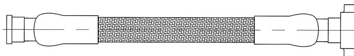
Przykład kompletacji przewodu ROTARY DRILLING DN75
