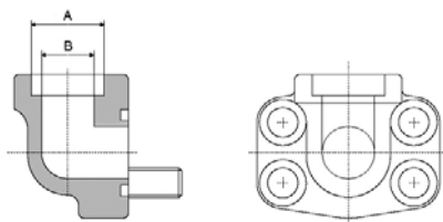
Przylączy kołnierzowe 90° SAE 3000 do wstawiania
