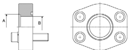
Przylączy kołnierzowe SAE 3000 do wstawiania
