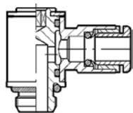
Przyłącze kątowe nastawne, gwint zewnętrzny, mosiądz
