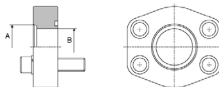
Przylączy kołnierzowe SAE 6000 do wstawiania
