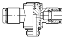
Przyłącze trójnik „T” nastawne, gwint zewnętrzny, mosiądz
