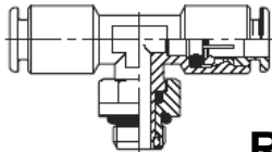
Przyłącze trójnik „T” obrotowy, gwint zewnętrzny
