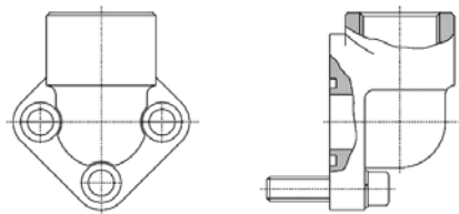
Przyłącze kołnierzowe 3-otworowe 90° / GW BSP
