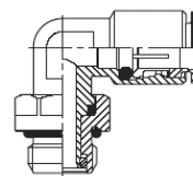
Przylącze kątowe obrotowe, gwint zewnętrzny
