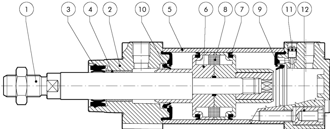
Budowa siłownika ISO 1552
